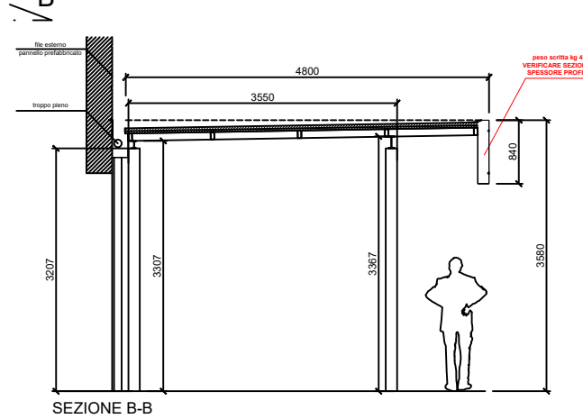
SEZIONE B-B
