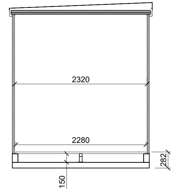
SEZIONE BOX
