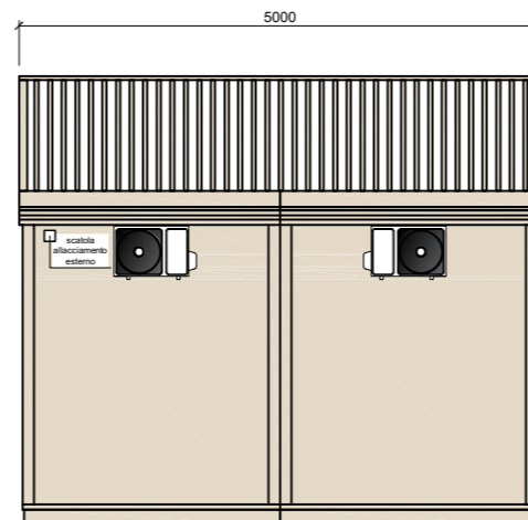
PROSPETTO LATERALE DX
