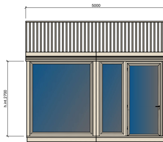
PROSPETTO LATERALE SX
