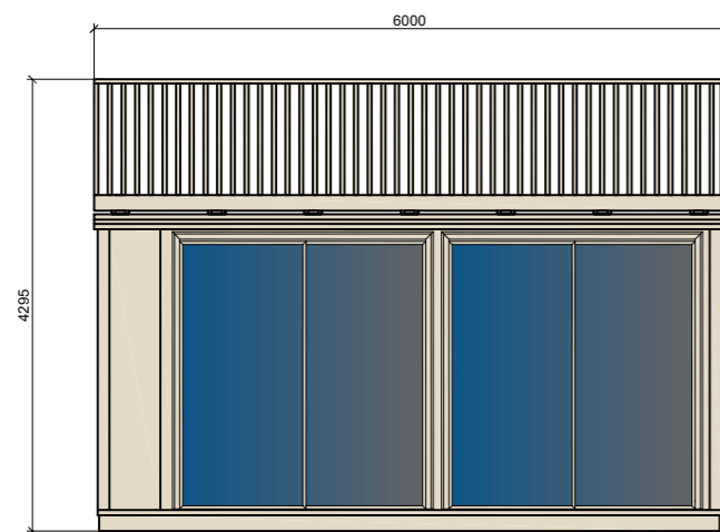
PROSPETTO FRONTALE
