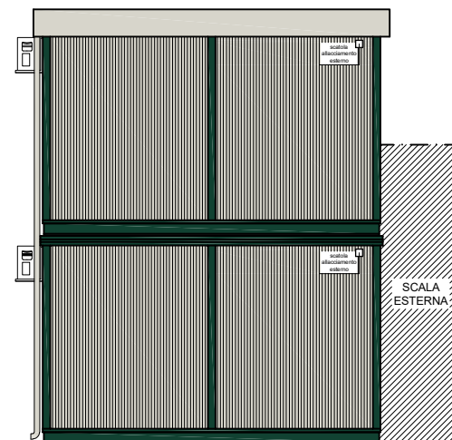
PROSPETTO POSTERIORO RIBALTATO DI 180°
