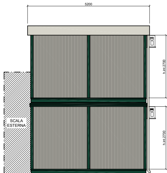
PROSPETTO FRONTALE
