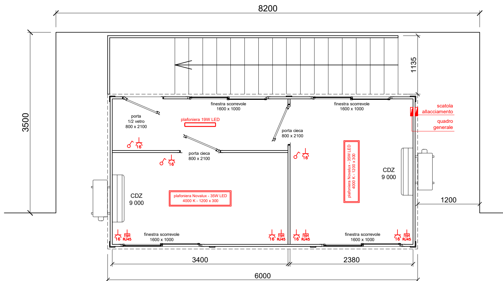
PIANO PRIMO
