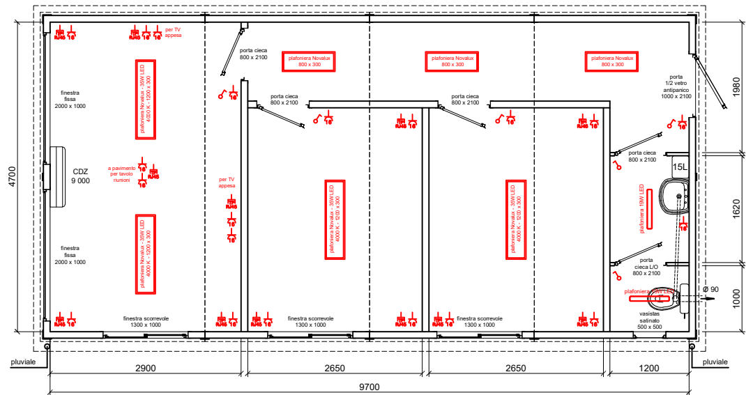
PIANO PRIMO
